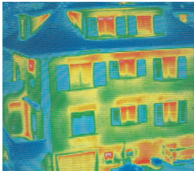
Bild mit 1-fach-Verglasung (hoher Energieverlust)
