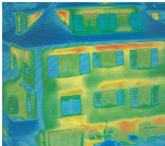
Bild mit rekord-Wärmeschutzverglasung (geringer Energieverlust)
